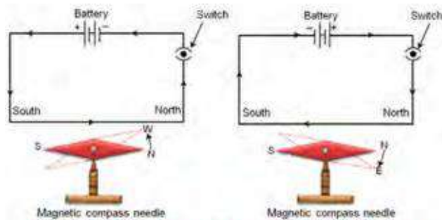
चित्र 11.8 विद्युत् करेन्टको दिशासँगै चुम्बकीय कम्पासको निडिलले देखाउने तारको दिशा
