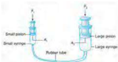
चित्र ४.११ हाइड्रोलिक मेसिनको नमूना निर्माण
