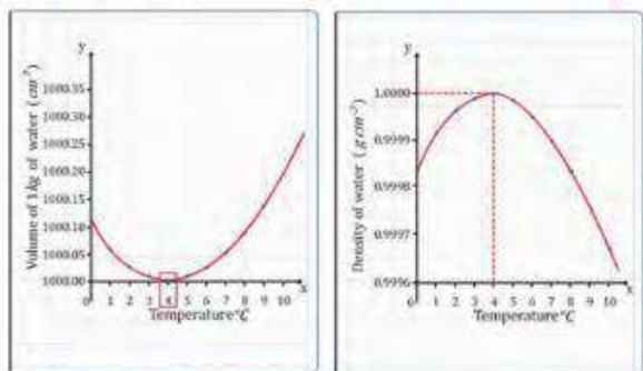
चित्र 9.4 पानीको आयतन र घनत्व तथा घनत्व र तापक्रमद्विचको सम्बन्ध
