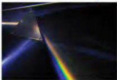
चित्र 10.41 प्रिज्मबाट प्रकाशको विच्छेदन
