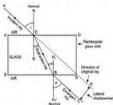
चित्र 10.9 काँचको स्ल्याबबाट प्रकाशको आवर्तन
