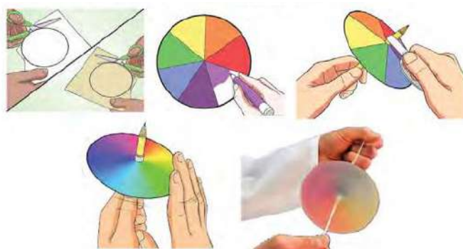
चित्र 10.42 न्युटनको चक्का (Newton's disc) निर्माण
