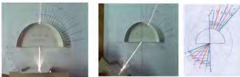
चित्र 10.10 अर्धवृत्ताकार काँचको स्ल्याबबाट प्रकाशको आवर्तन
